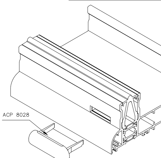
SOLUZIONE PER DRENAGGI TIPO 2
